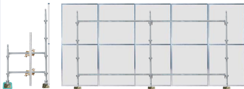
クサビ足場
