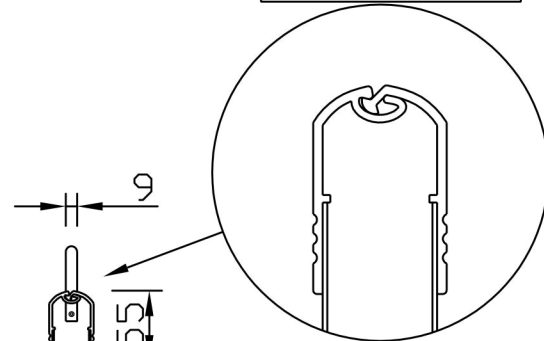
屋根部拡大断面図
