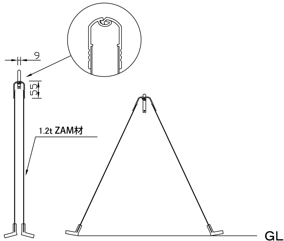
屋根部 拡大断面図
